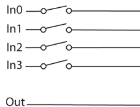
4:1 Multiplexer
